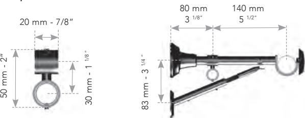
Colliers adaptateurs Ø 19 mm pour supports mur - Ø 3/4" Adapters for wall brackets
